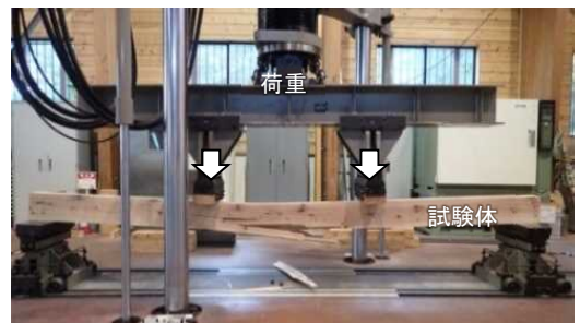
曲げ試験の実施状況
